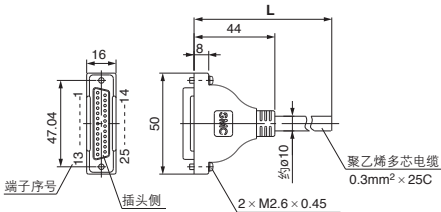
D型辅助插头电缆组件 各端子序号线色表
