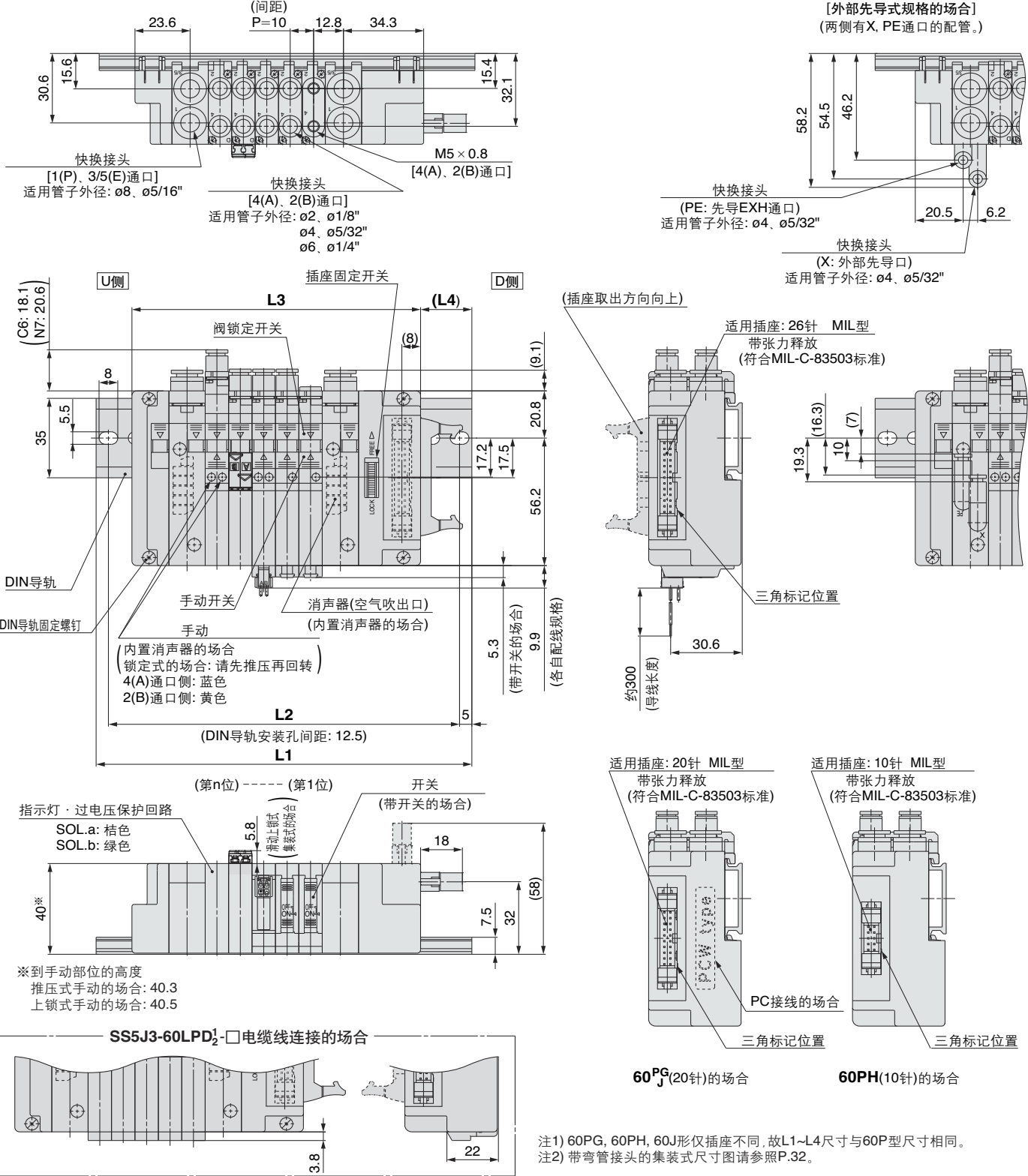
L: 尺寸表
