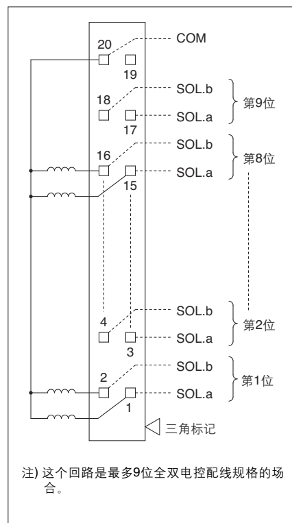
60LPG型扁平电缆插座(20针)
