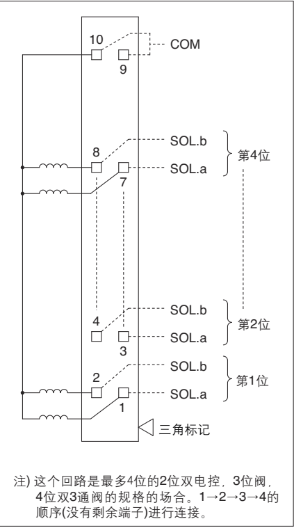
60PH型扁平电缆插座(10针)
