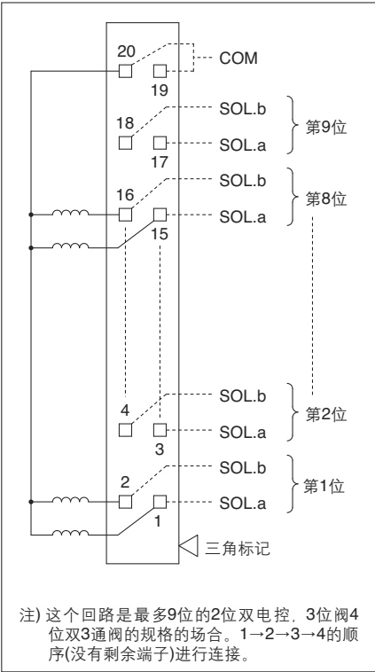
60J型扁平电缆插座(20针 PC接线)
