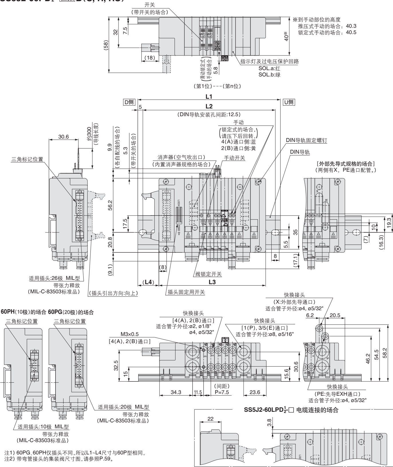
L : 尺寸表
