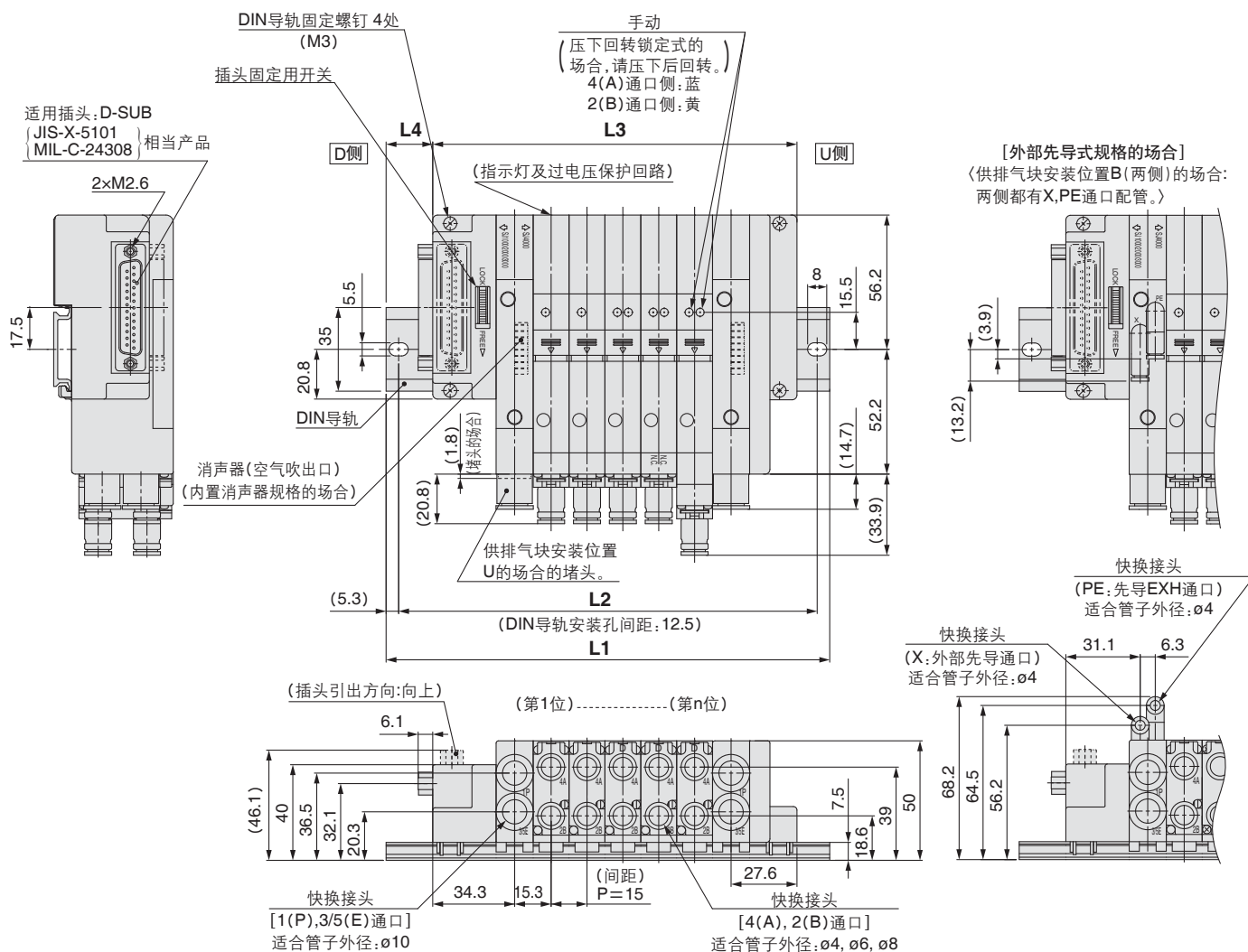
L : 尺寸表
