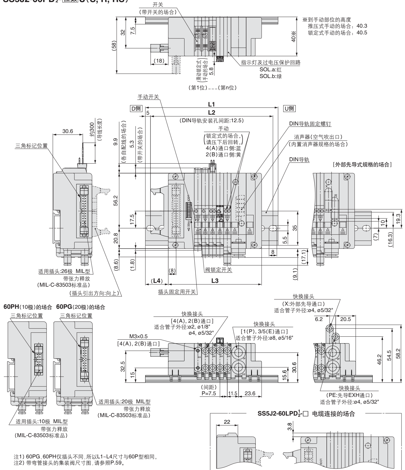
L : 尺寸表
