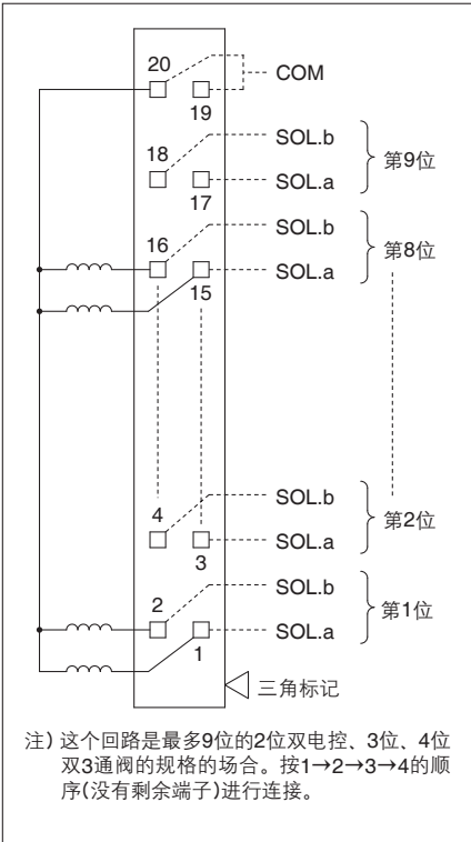
60PG型扁平电缆插头(20极)
