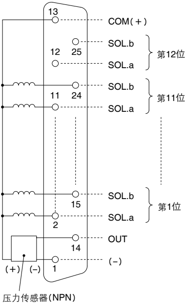
D型辅助插头型(25极)
