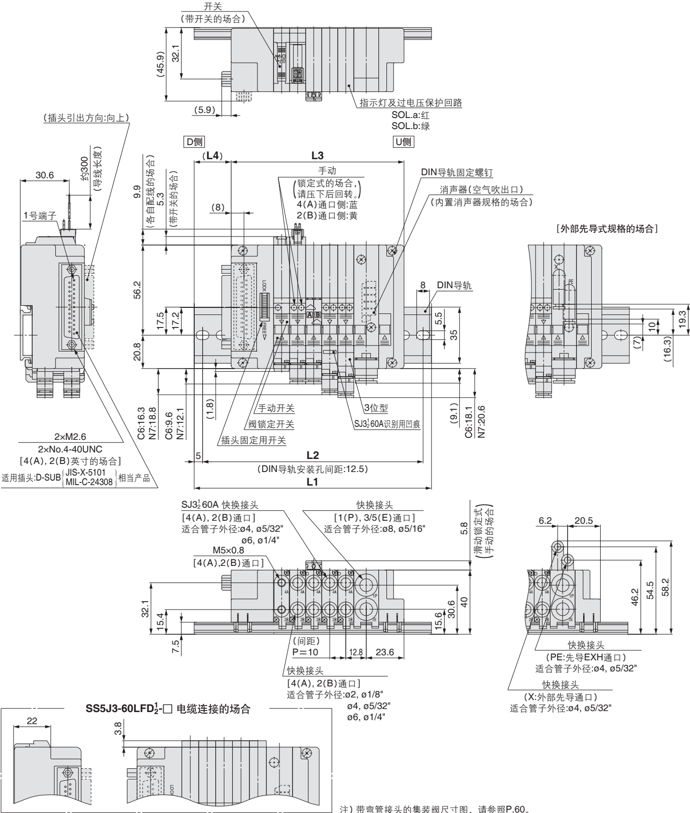
L : 尺寸表
