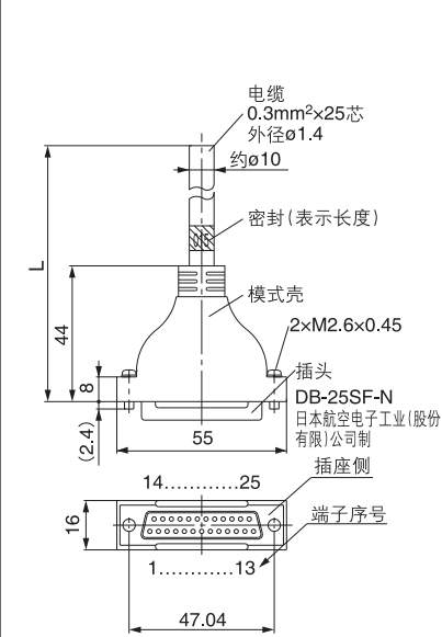
D型辅助插头电缆组件
