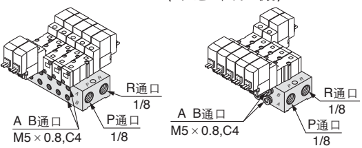
S32型 (单电控的先导阀与A,B通口在同一侧。)
