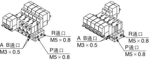
S31型 (单电控的先导阀与A,B通口在同一侧。)
