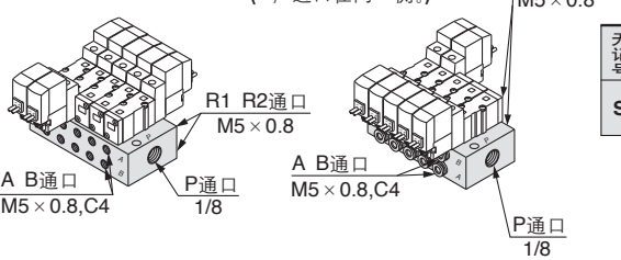
S46型 (单电控的先导阀与A,B通口在同一侧。)
