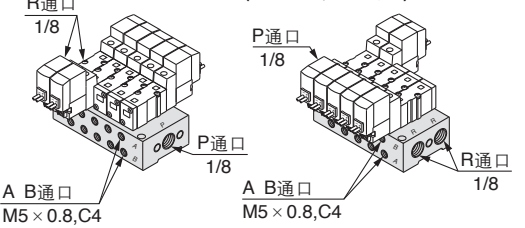
S41型 (单电控的先导阀与A,B通口在同一侧。)
