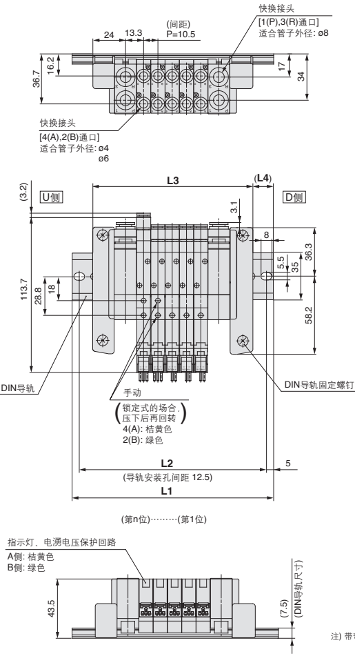
内部先导式集装式 L : 尺寸表
