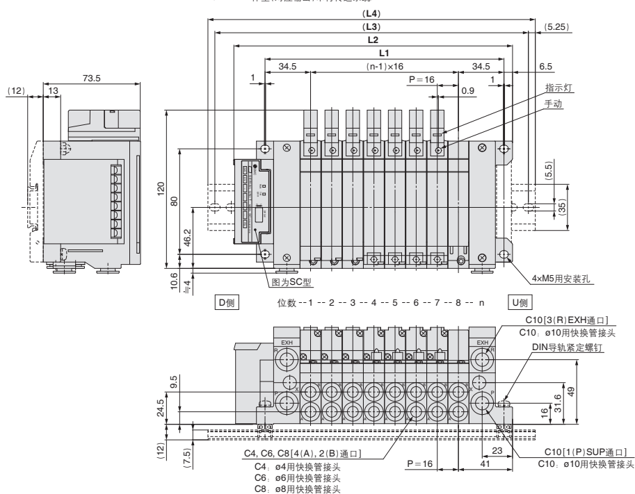
耐尘・防喷流型 (IP65) SI单元 <EX124—体型 (对应输出) 串行传送系统>
