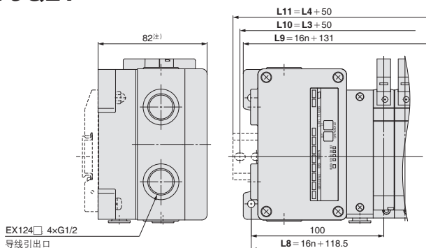
耐尘・防喷流型 (IP65) SI单元 <EX124—体型 (对应输出) 串行传送系统>
