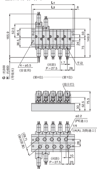
L：尺寸表
